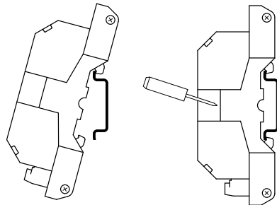
Abb. 1: Einbau
