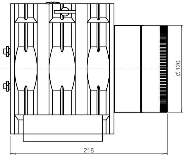
Option OP-06 (monté avec bride d'adaptation pour codeur Ø58 à axe Ø6)
