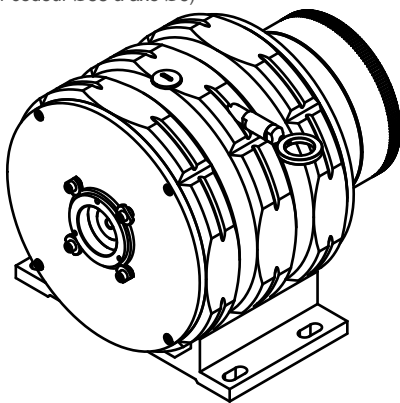
Option OP-06 (monté avec bride d'adaptation pour codeur Ø58 à axe Ø6)
