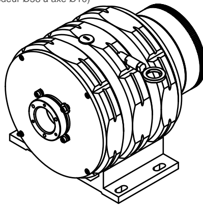
Option OP-10 (monté avec bride d'adaptation pour codeur Ø58 à axe Ø10)
