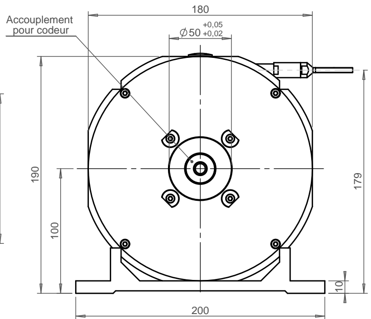
Option OP-12 (monté avec bride d'adaptation pour codeur Ø90 à axe Ø12)
